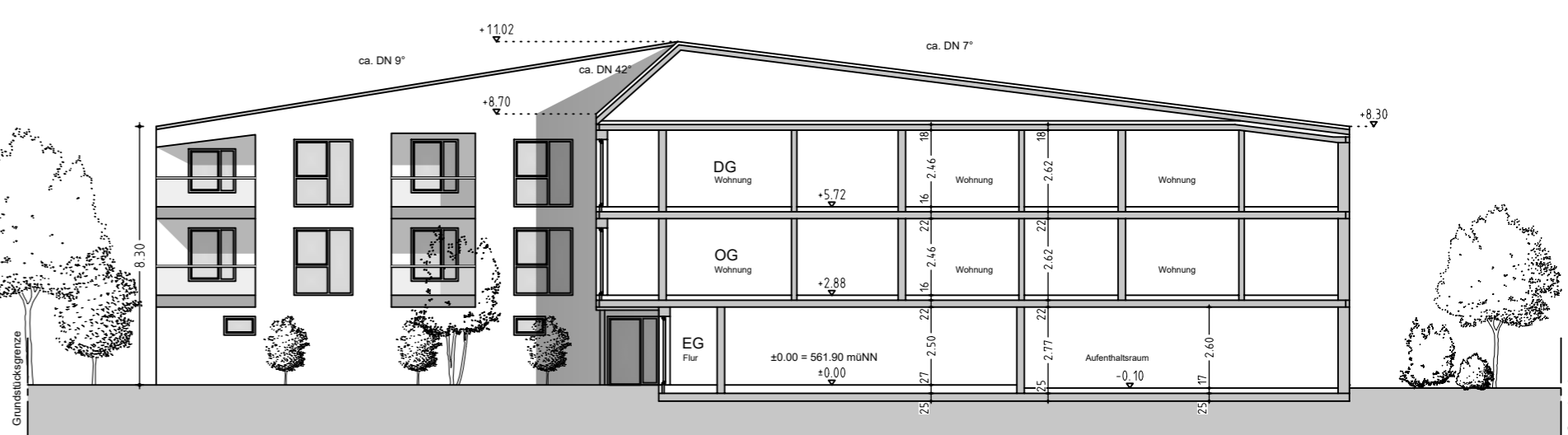
Schnitt I-I
